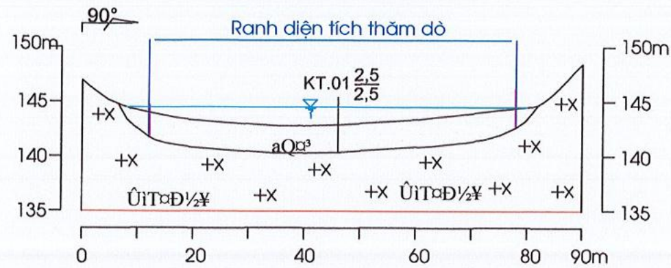
MẶT CẮT TUYẾN T1
