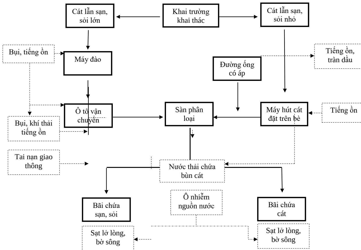
Hình 1. 2: Sơ đồ công nghệ khai thác và dòng phát thải Thuyết minh công nghệ khai thác:
