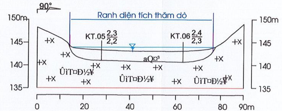
MẶT CẮT TUYẾN T4
